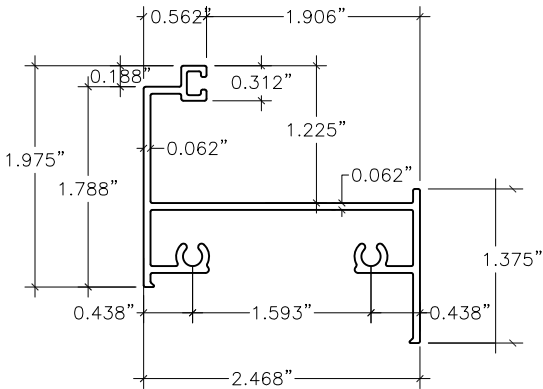
2 FRAME JAMB
